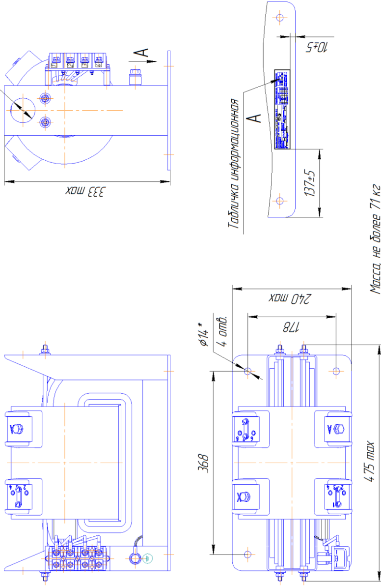
Рисунок А.1 – Габаритные, установочные, присоединительные размеры и масса трансформаторов ОЛС-НТЗ-5,0/6(10)
