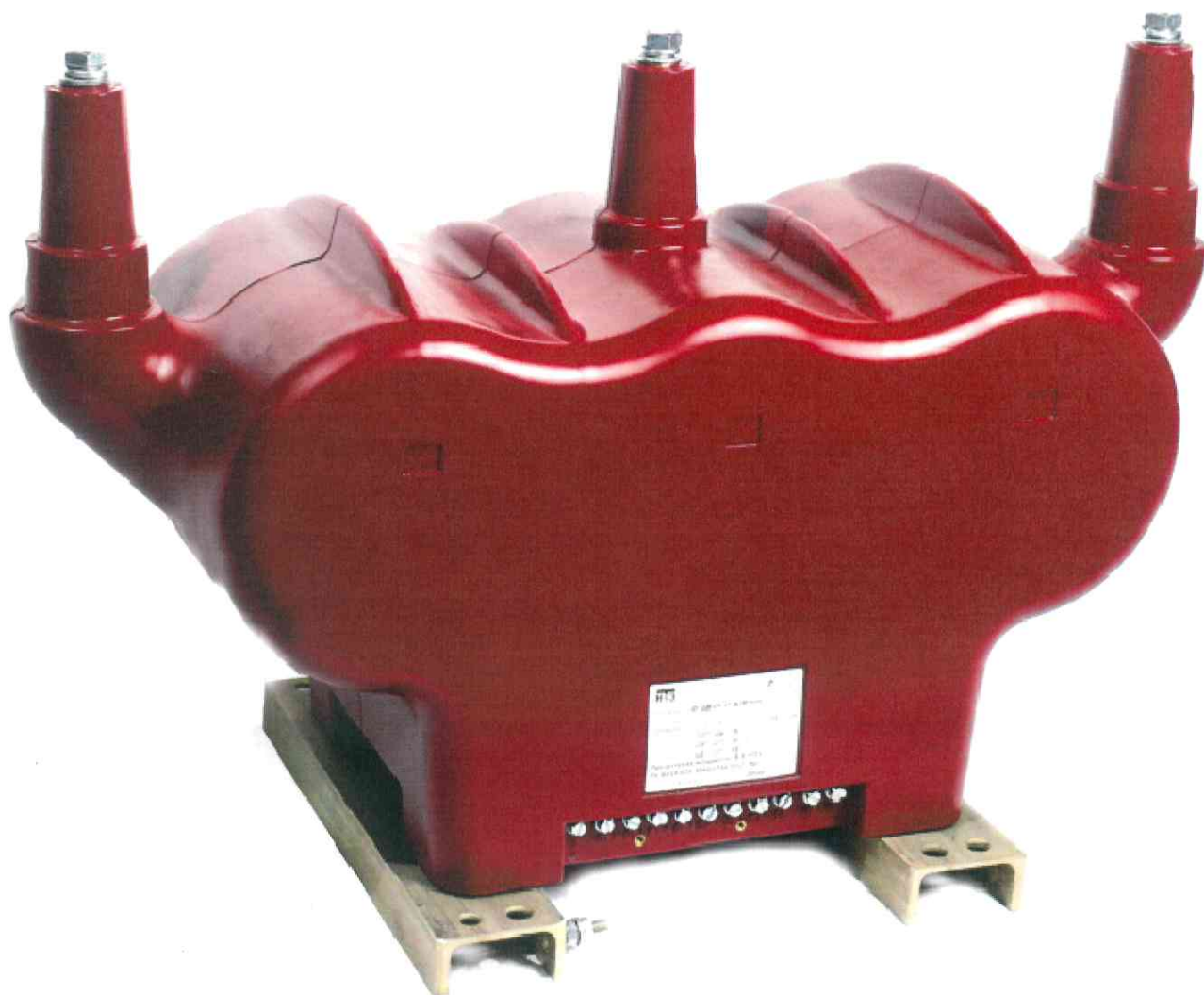
Рисунок 2 – Общий вид трансформаторов напряжения антирезонансных трехфазных НАЛИ-НТЗ-20(35)
