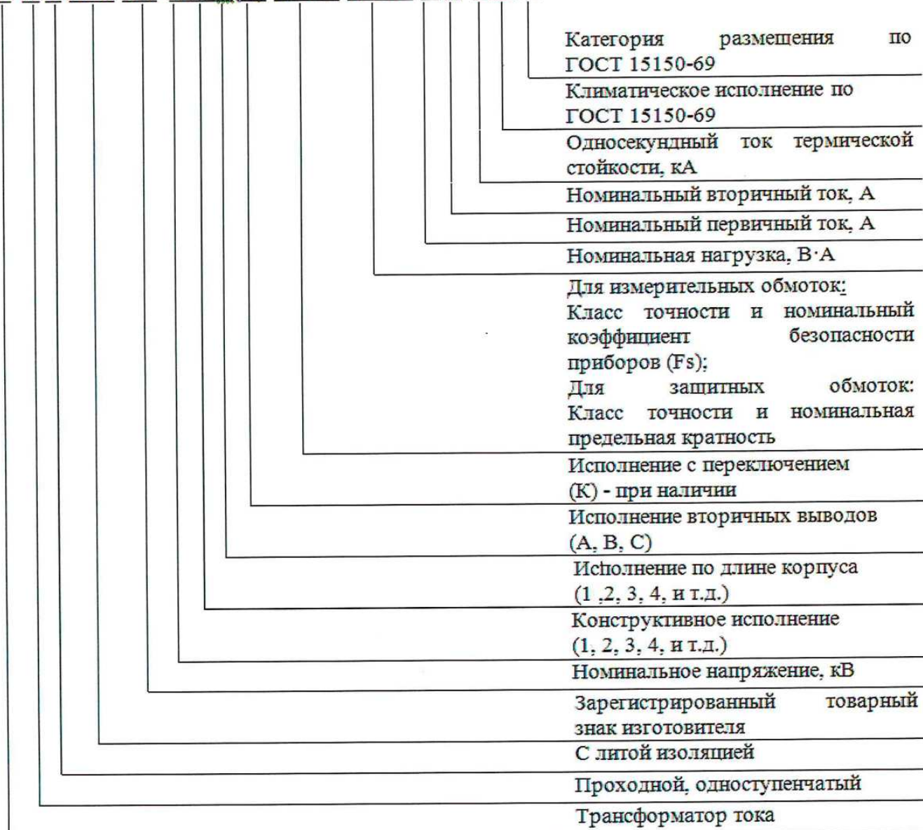
Рисунок 2 - Структура условного обозначения трансформаторов тока ТПЛ-НТЗ
