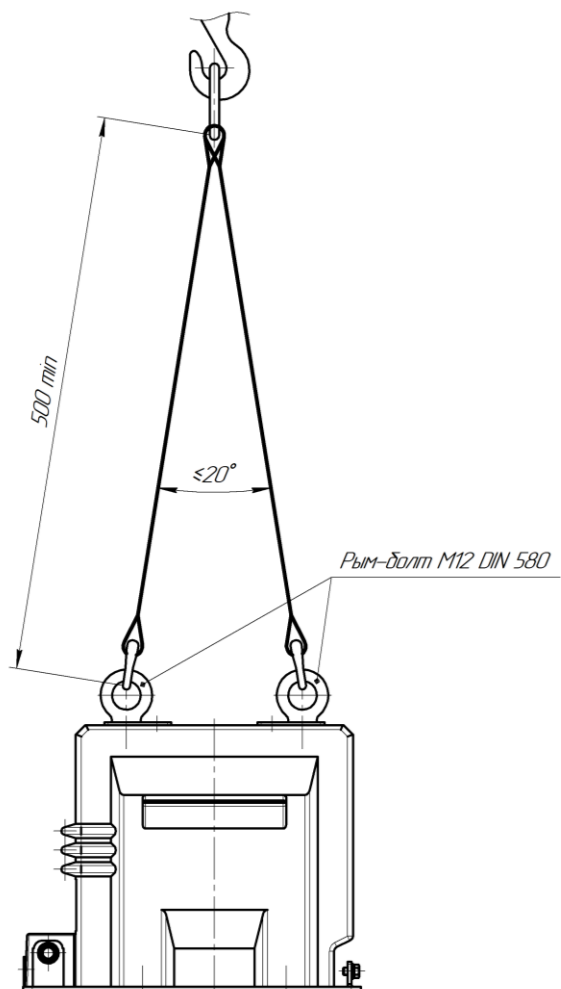
Рисунок Г.2 – Схема строповки трансформаторов ТОЛ-НТЗ-20-81Е
