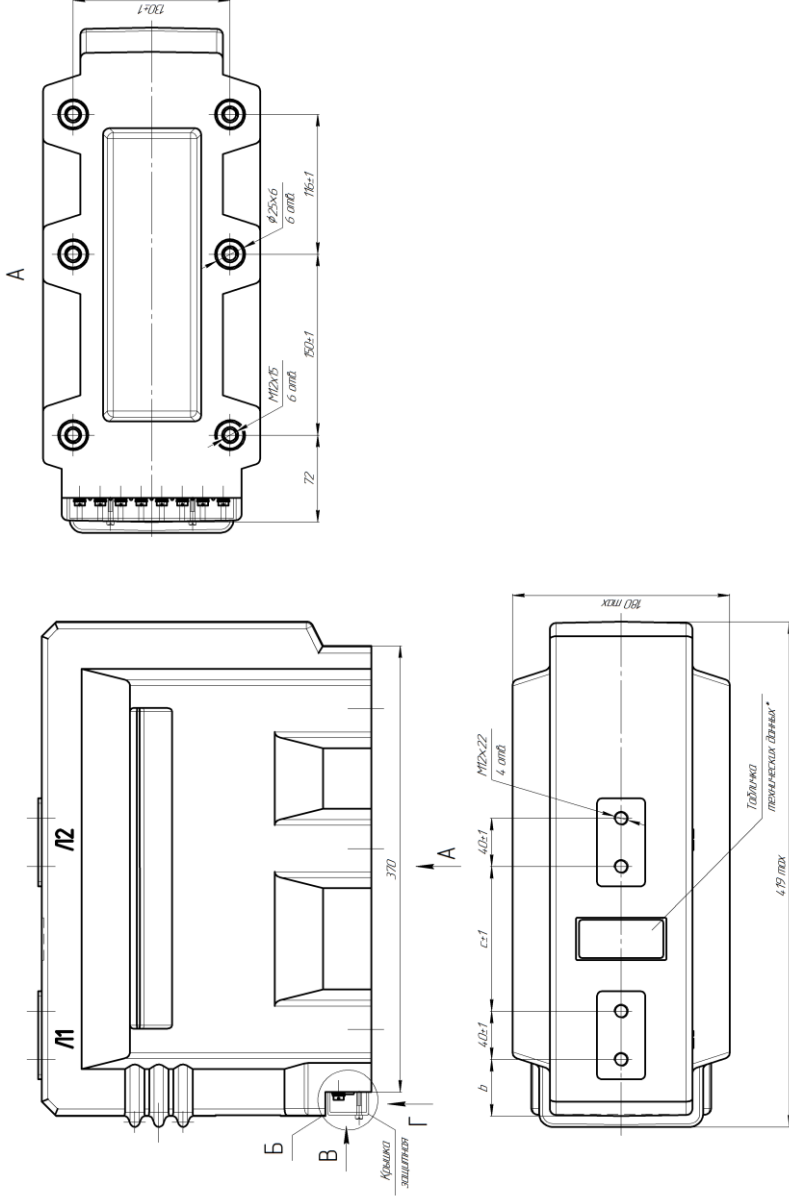
Рисунок А.3 — Габаритные, установочные, присоединительные размеры трансформаторов ТОЛ-НТЗ-20-13
