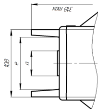
Рисунок А.2 – Габаритные, установочные, присоединительные размеры трансформаторов ТОЛ-НТЗ-20-11, -13
