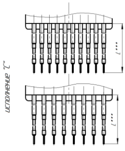
Рисунок А.5 – Варианты исполнения вторичных выводов ТЛН-НТЗ-20-11, -13
