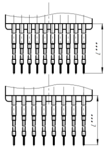
Рисунок А.5 – Варианты исполнения вторичных выводов ТОЛ-НТЗ-20-11, -13
