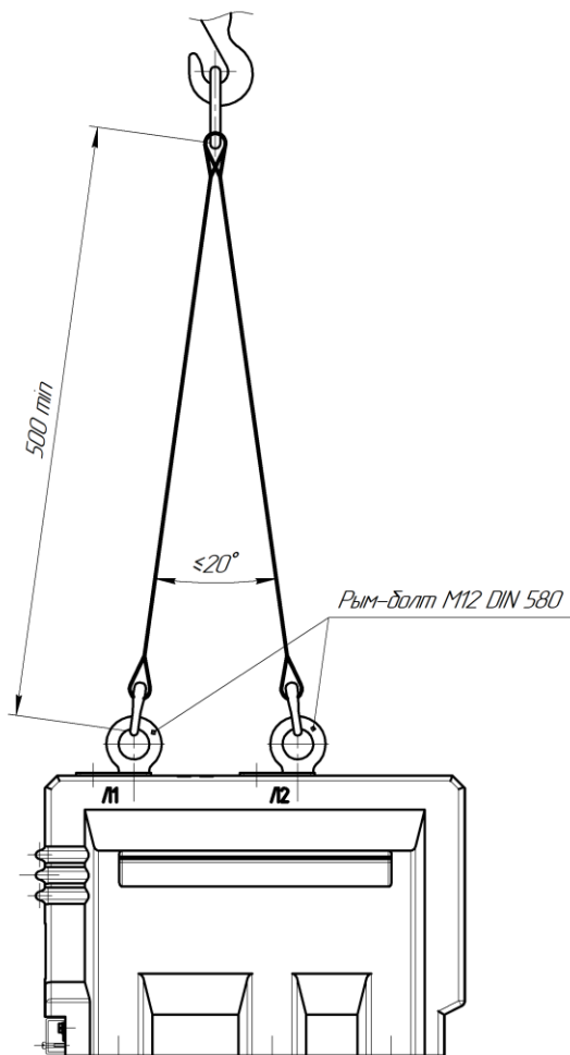
Рисунок Г.1 – Схема строповки трансформаторов ТОЛ-НТЗ-20-11, -13
