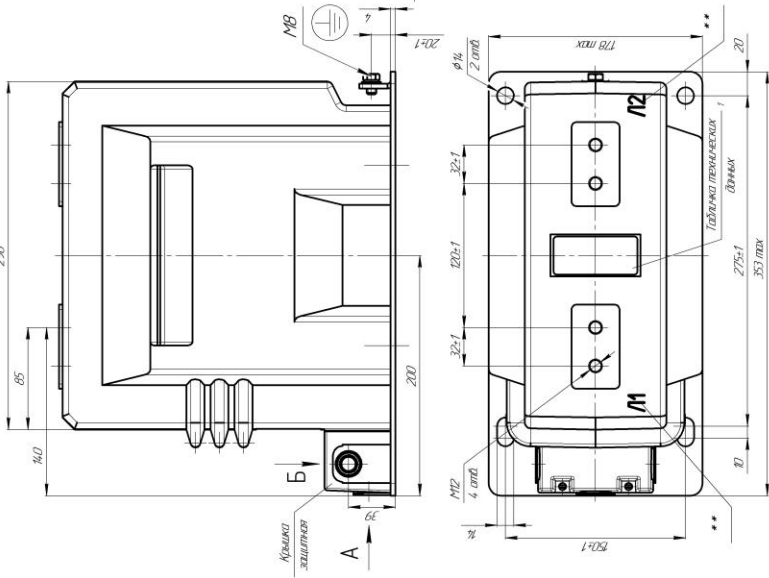
Рисунок А.6 – Габаритные, установочные, присоединительные размеры и масса трансформаторов ТОЛ-НТЗ-20-81Е
