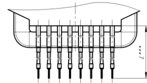
Рисунок А.6 – Варианты исполнения вторичных выводов ТОЛ-НТЗ-35-11, -12
