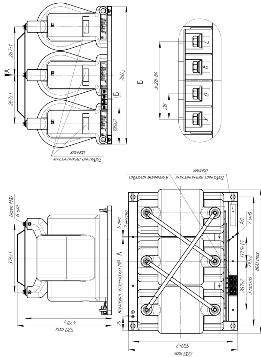
Масса трансформатора, не более, 360 кг Рисунок А.1 – Габаритные, установочные, присоединительные размеры и масса трансформаторов ТЛС-НТЗ-40/6(10), Д/Ун-11
