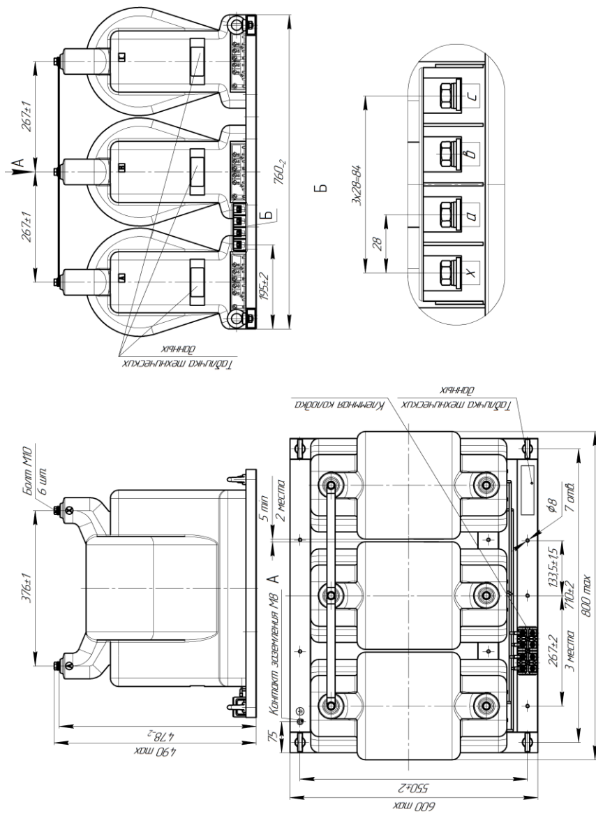
Рисунок А.2 – Габаритные, установочные, присоединительные размеры и масса трансформаторов ТЛС-НТЗ-40/6(10), У/Ун-0 Масса трансформатора, не более, 360 кг
