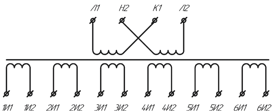
Рисунок Б.5 – Схема электрическая принципиальная для исполнений «П» (переключение по первичной стороне) ТОЛ-НТЗ-35-IV-12
