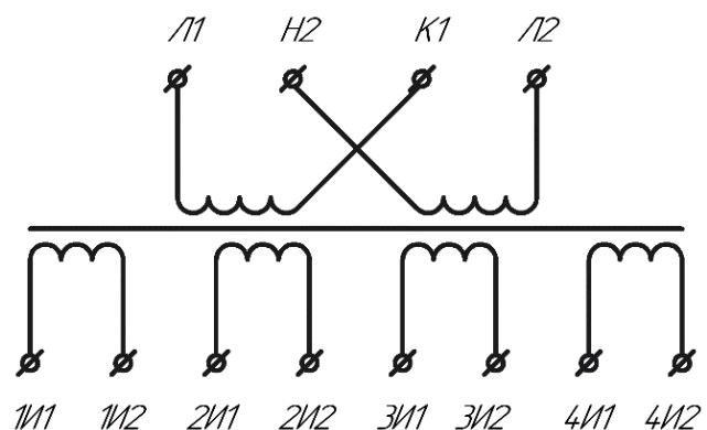
Рисунок Б.2 – Схема электрическая принципиальная для исполнений «П» (переключение по первичной стороне) ТОЛ-НТЗ-35-IV-11
