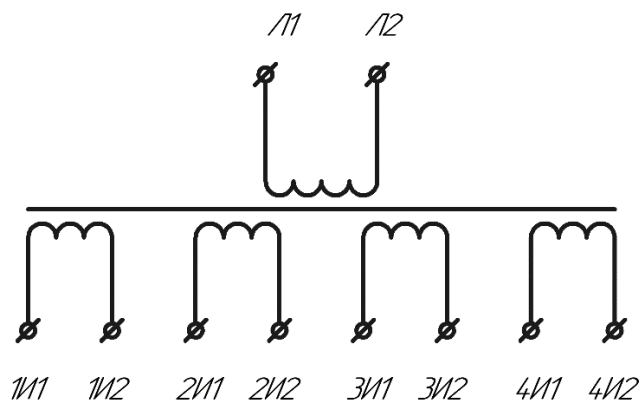
Рисунок Б.1 – Схема электрическая принципиальная для стандартных исполнений ТОЛ-НТЗ-35-IV-11
