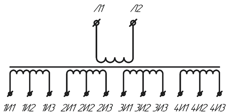
Рисунок Б.3 – Схема электрическая принципиальная для исполнений «К» (с ответвлениями на вторичных обмотках) ТОЛ-НТЗ-35-IV-11
