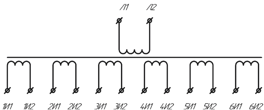
Рисунок Б.4 – Схема электрическая принципиальная для стандартных исполнений ТОЛ-НТЗ-35-IV-12 и ТОЛ-НТЗ-35-IV-21
