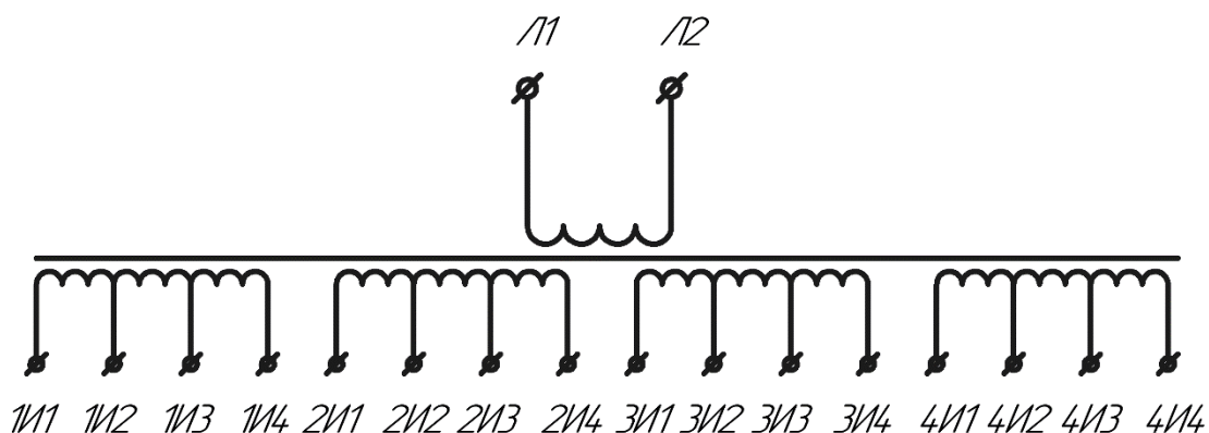
Рисунок Б.6 – Схема электрическая принципиальная для исполнений «К» (с ответвлениями на вторичных обмотках) ТОЛ-НТЗ-35-IV-12 и ТОЛ-НТЗ-35-IV-21
